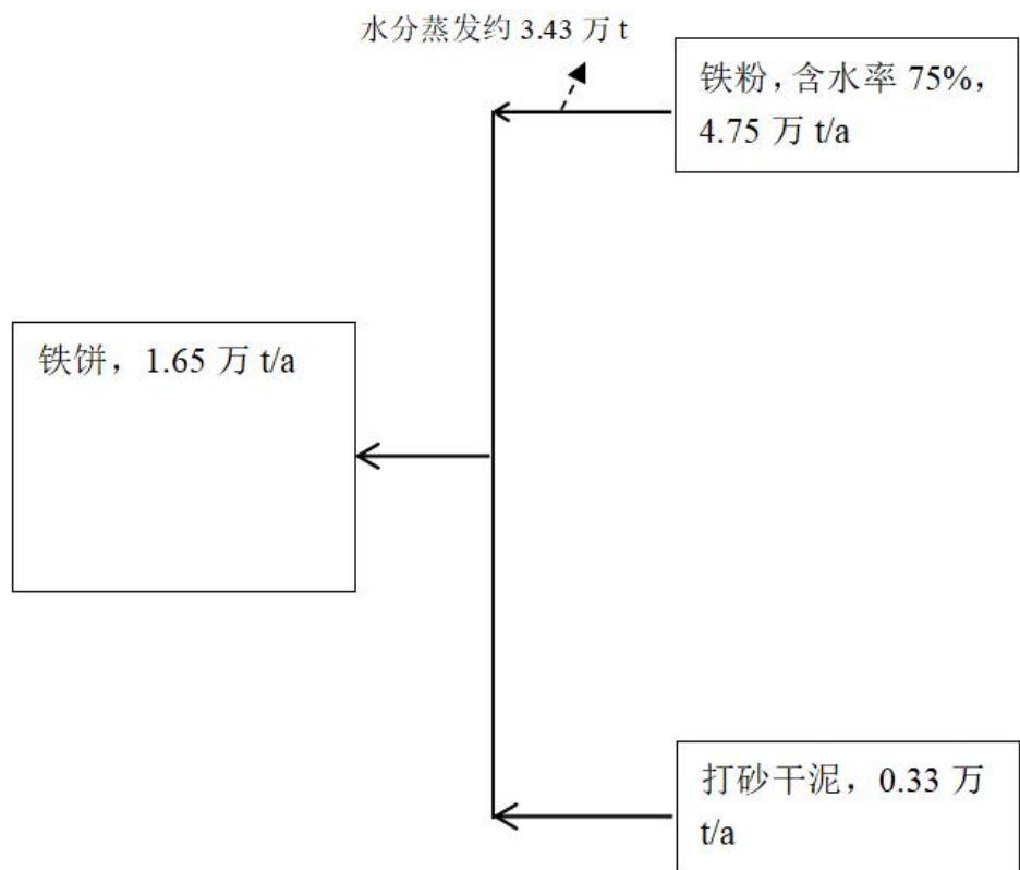
图 1 物料平衡图
